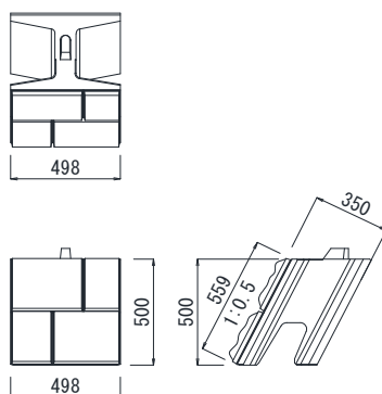
規格諸元
