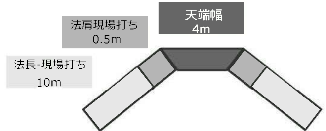
天端部現場打ちコンクリート被覆工施工体制
